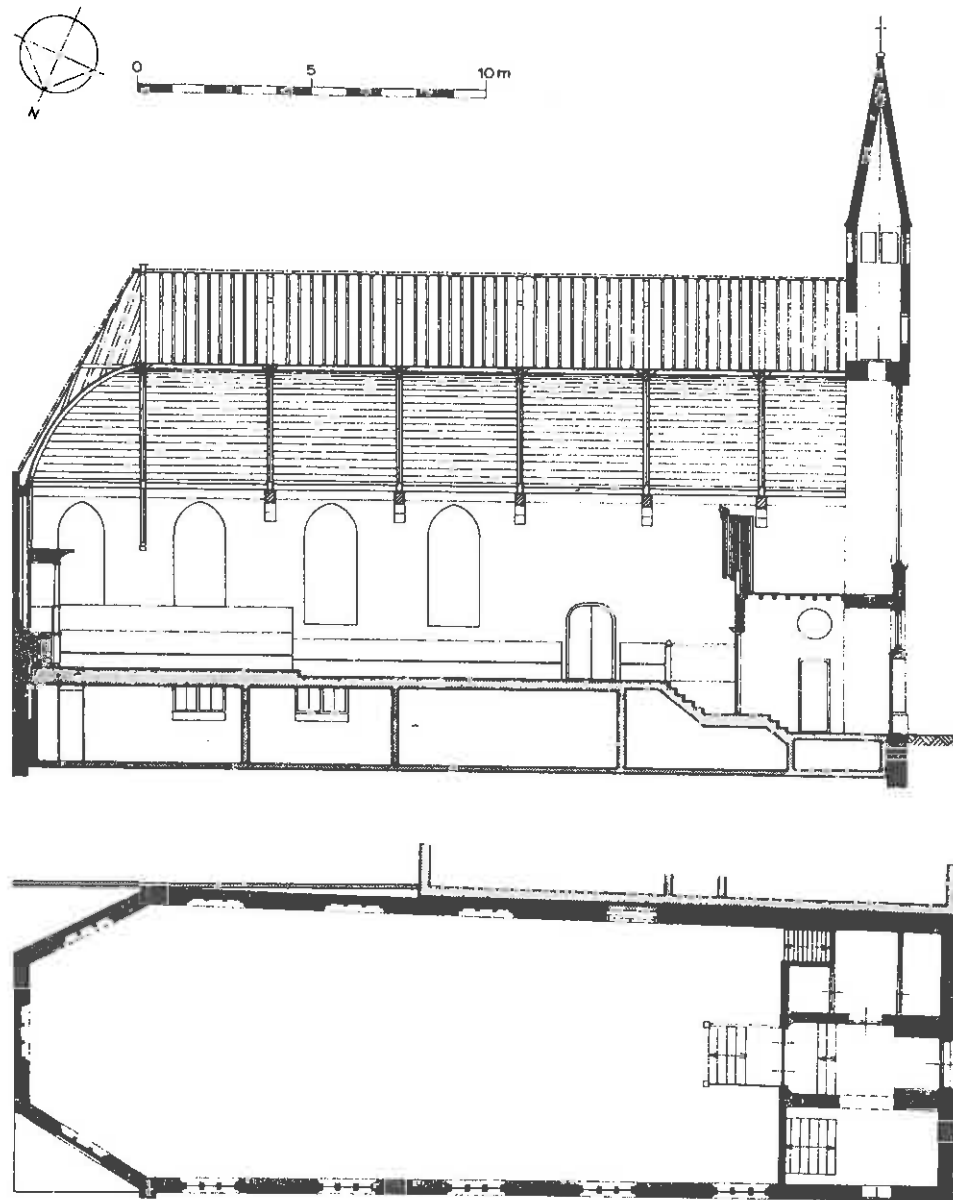
Langsdoorsnede en plattegrond 1978.
